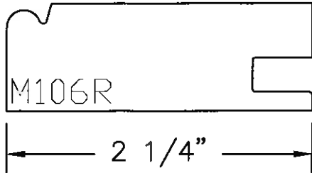
Door Profile
