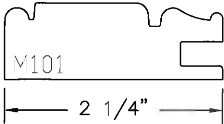
Door Profile
