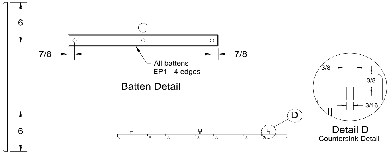
SLAB DOOR (SD)
