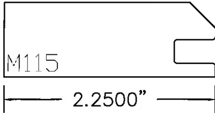
Door Profile
