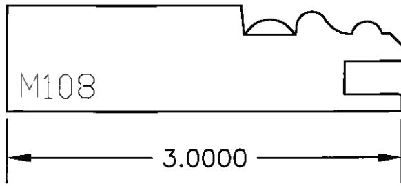
Door Profile
